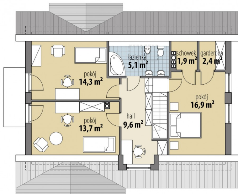
PODDASZE
