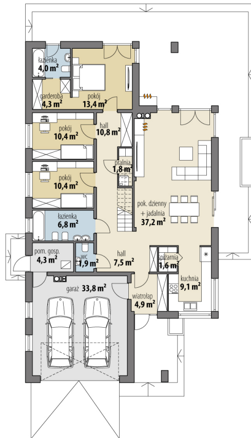
RZUT PARTER
