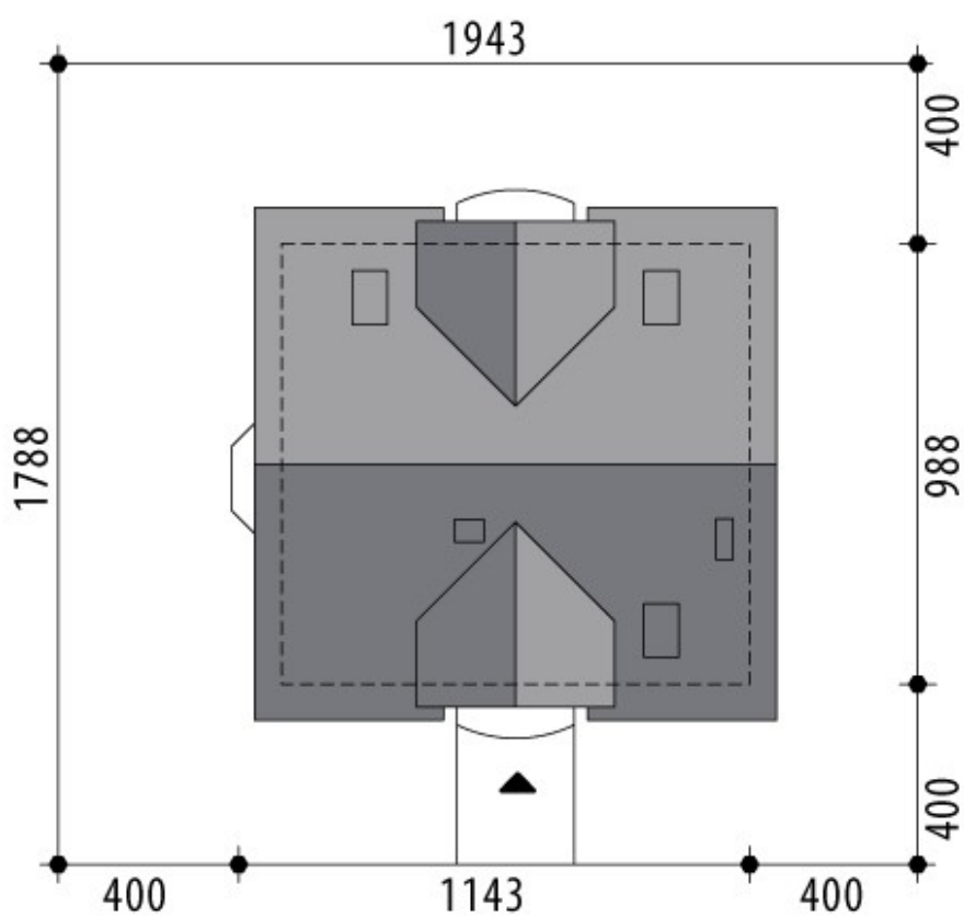
SYTUACJA
