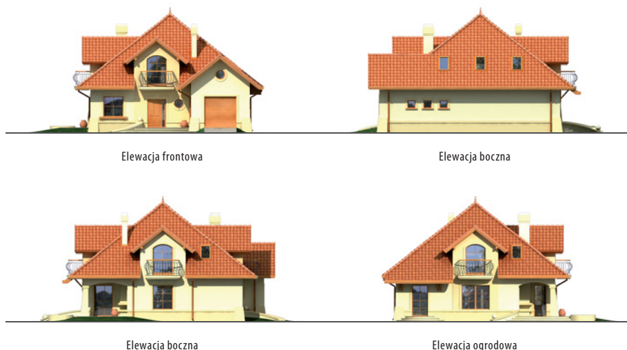
Elewacja boczna
