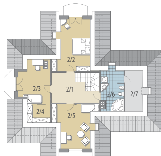
Poddasze
