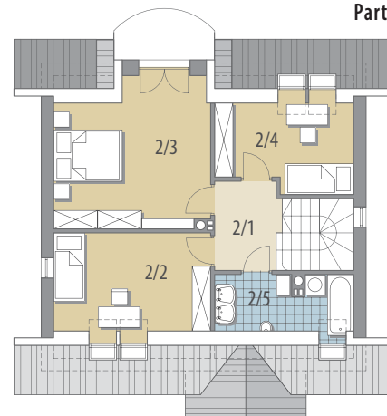
Poddasze
